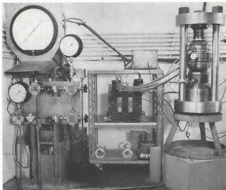
Fig. 2. — Appareil haute pression à pistons profilés avec, à gauche, les dispositifs de commande et de contrôle (phot. X).
